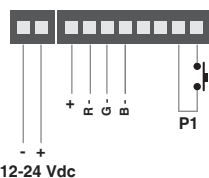
RGB
